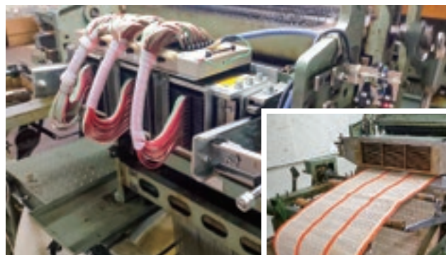
導入した紋紙不要の「ダイレクトジャガード」 (右下は従来のジャガード織機)
